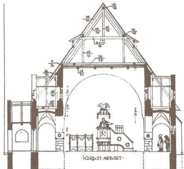
A „kakasos” templom tervrajza
